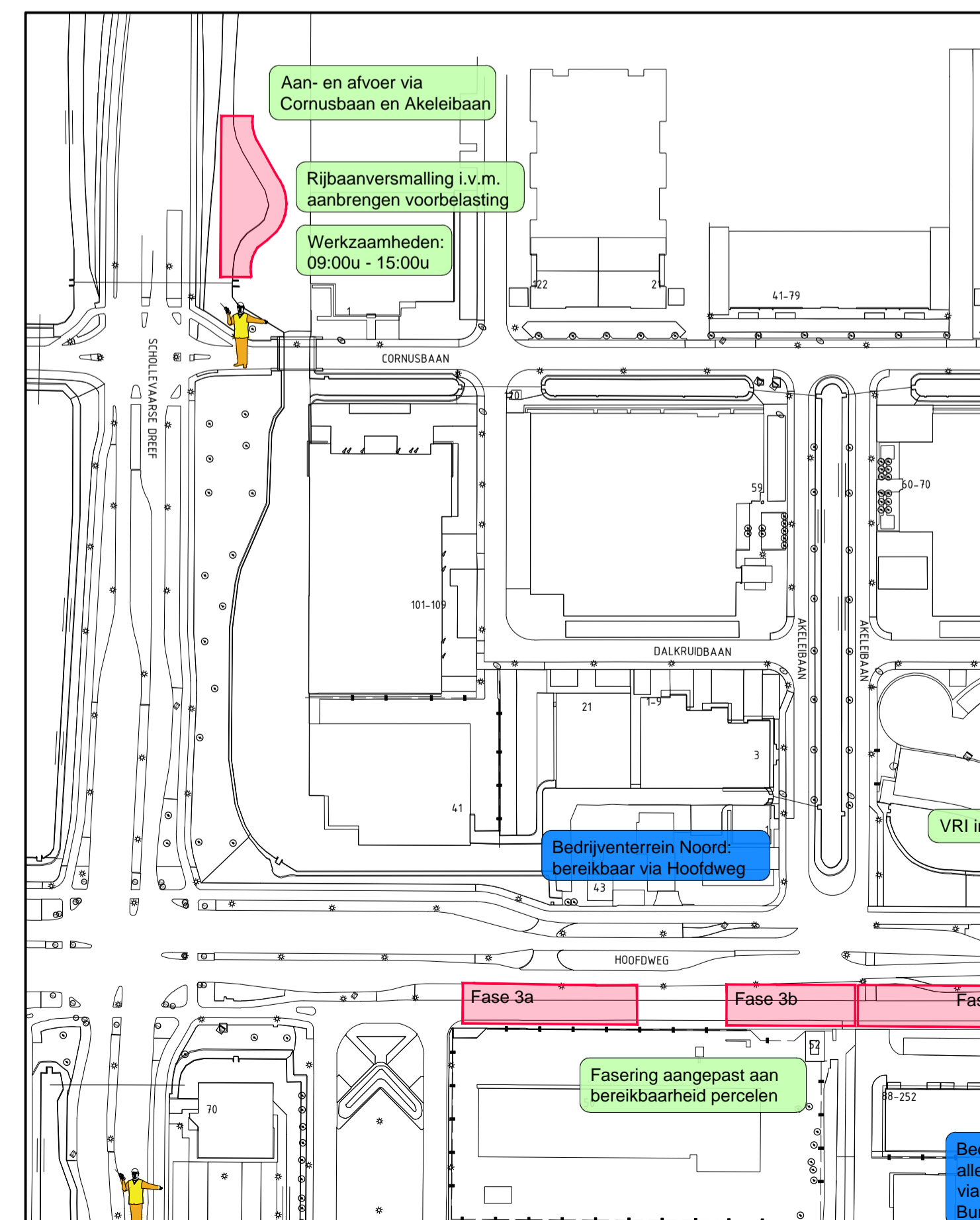
Fase 3: Aanpassingen secundaire weg (inclusief aanpassen watrgang Cornusbaan en laatste slag voorbelasting Britse Zoom) -> Uitvoeringstijd 3 weken
